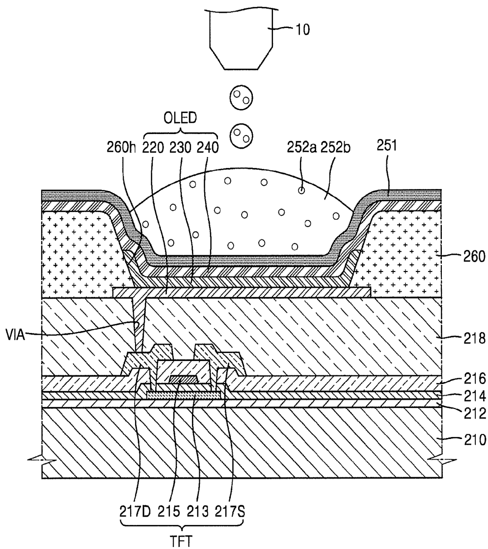
FIG. 3F
